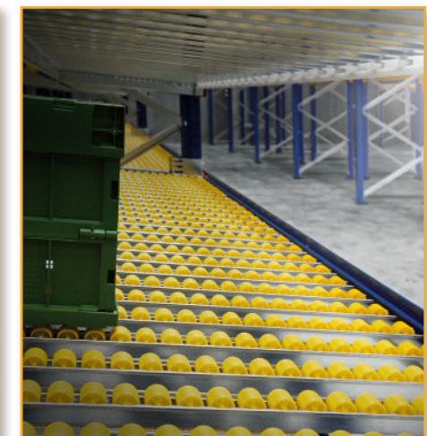
Σύστημα κυλιόμενων ραφιών για χρήση Picking
